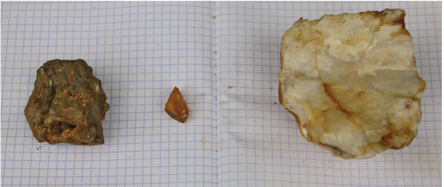
Fig. 7. Blocs et cristaux de quartz provenant du remblais au pied du Trou Madot, montrant une diversité d'aspects, de couleurs et de tailles de cristaux alors qu'ils proviennent de la même veine.
