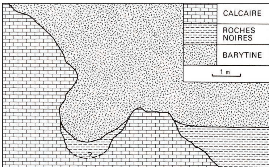
Fig. 5. Gisement de Fleurus : schéma de petite poche karstique remplie de minerais (reproduction de la fig. 5 de Dejonghe, 1989).
