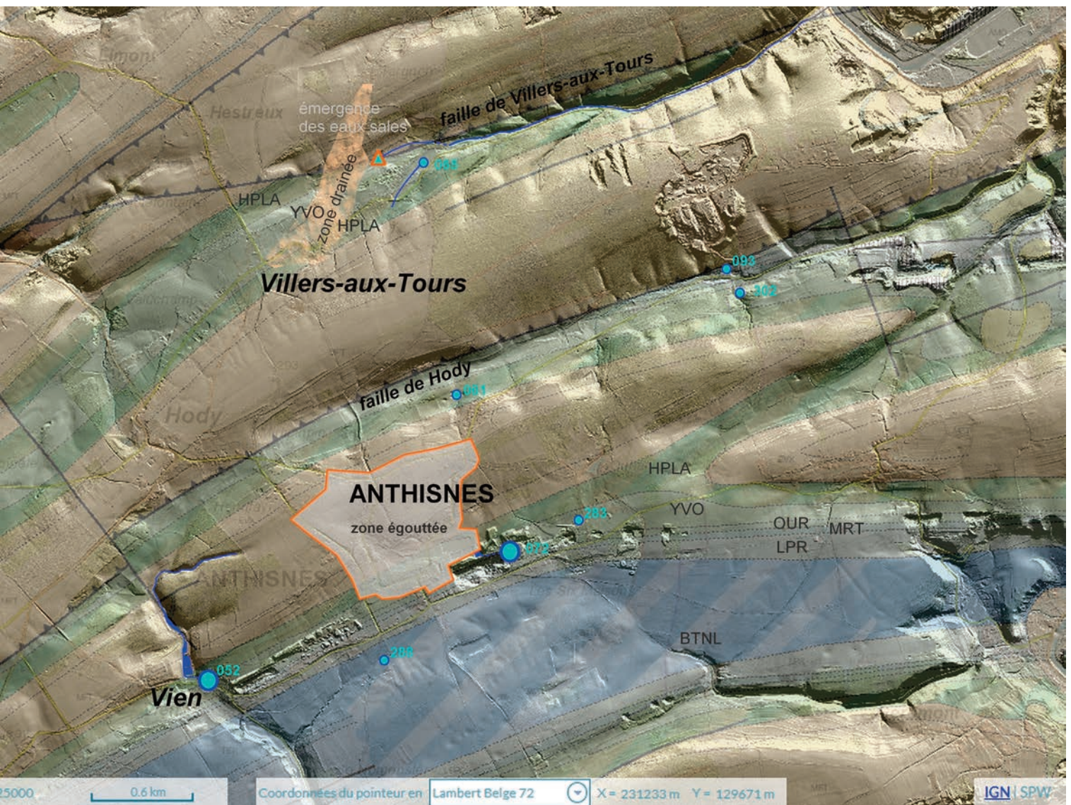
Fig. 2. Carte géologique, hydrogéologique et morphologique d'Anthignes – Ronds bleus : points de perte connus avec numérotation AKWA. Au 072, point d'absorption des égouts d'Anthignes (source : Walonmap).
