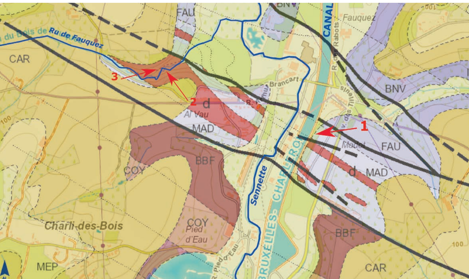
Fig. 2. Extrait de la carte géologique 39/5-6 (Braine-le-Comte, Feluy) révisée par Hennebert et Eggermont et publié par le SPW en 2002. Des complexes de roches appartenant à la fin de l'Ordovicien et au Silurien (massif du Brabant) présentent des intercalations volcaniques qui affleurent dans les vallées (Sennette & ru du Bois de Fauquez) et sur le versant où l'érosion a décapé la couverture de sables tertiaires. 1 : Grotte Madot le long du RAVeL en bordure du Canal Bruxelles-Charleroi. 2. & 3 : Affleurements de laves et tufs volcaniques dans le Bois des Roc.
