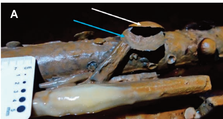
Fig. 3. IRSS se développant sur la barrière longeant le chemin de halage du tunnel de Godarville. (A) IRSS de plus de 2 cm de large dont les deux « coques » sont ouvertes. La flèche blanche pointe la coque supérieure, la flèche bleue la coque inférieure. (B) Plusieurs IRSS de différents diamètres, « coques » fermées.
