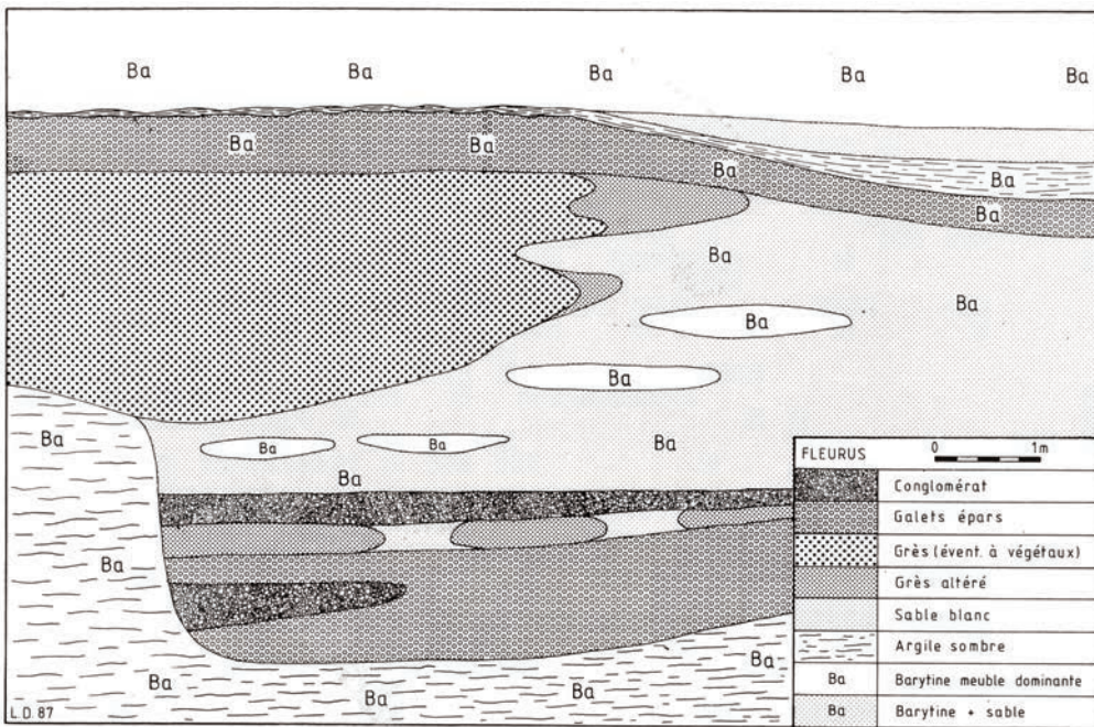
Fig. 7. Gisement de Fleurus. Cette coupe verticale nord-sud, à la partie orientale de l'exploitation, montre l'alternance tranchée de sédiments stériles et minéralisés (reproduction de la fig. 9 de Dejonghe, 1989). De bas en haut, on observe :
