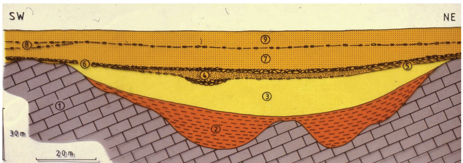
Fig. 4. Gisement de Fleurus coupe schématique NE- SW (reproduction de la figure 4 de Dejonghe, 1989)
